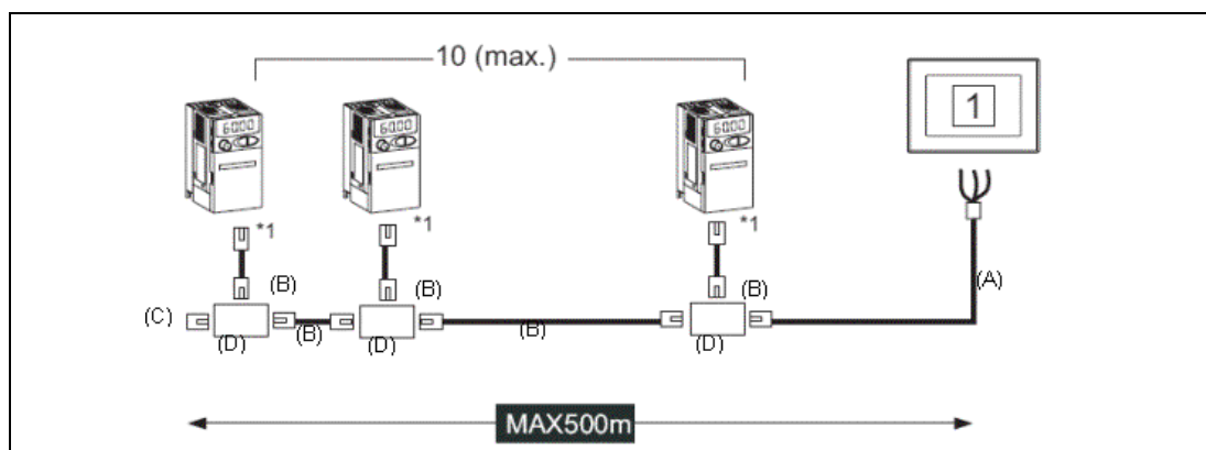
Рис. 2: Многоточечное соединение
